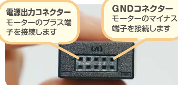
1 コネクターの接続箇所を確認する
